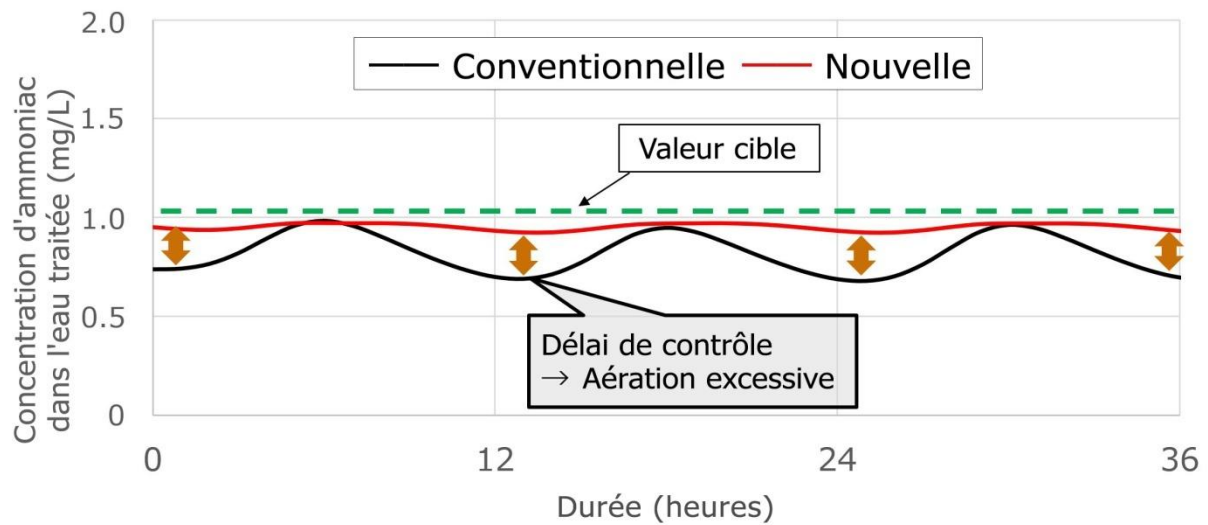
Fig. 2 Suppression de l'effet du délai de contrôle (résultats de la simulation)
